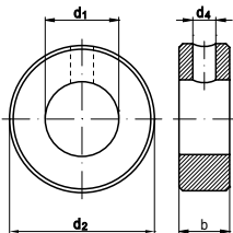
Form B = mit Bohrung für Korb- oder Kegelstift
